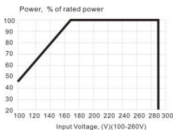
Diagramme de puissance/tension d'entrée
