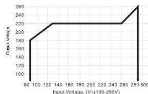
Diagramme de tension d'entrée/de sortie
