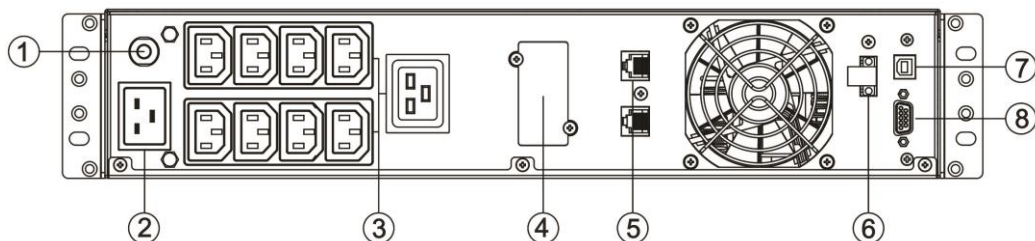
Schéma 2 : E3 Live 3000 VA – face arrière
