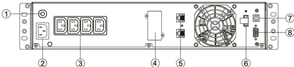
Schema 2: E3 Live 3000 VA – Rückwand
