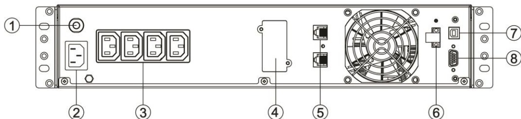
Schéma 2 : E3 Live 3000 VA – face arrière
