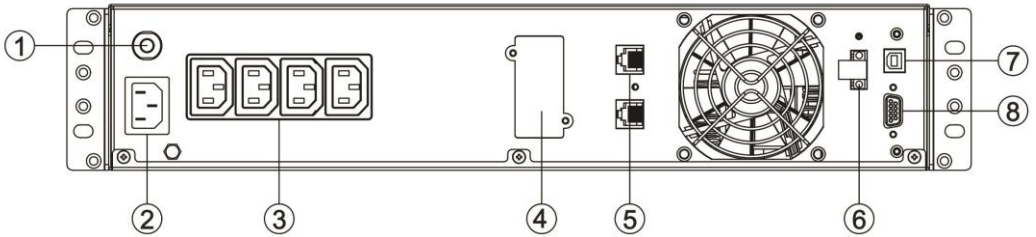
Schéma 2 : E3 Live 3000 VA – rear panel
