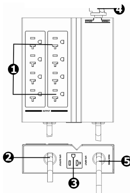
Prises NEMA
